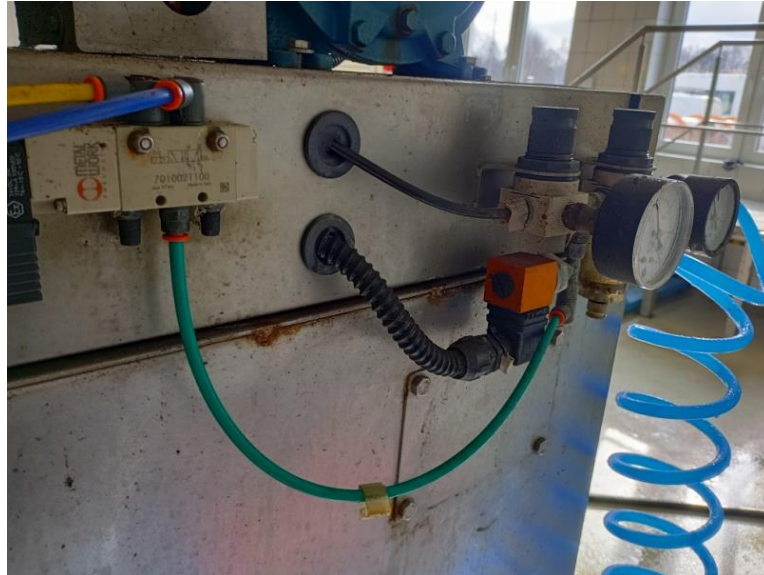
Układ pneumatyczny prasy taśmowej Monobelt podczas pracy urządzenia, z manometrami wskazującymi ciśnienie robocze układu.
