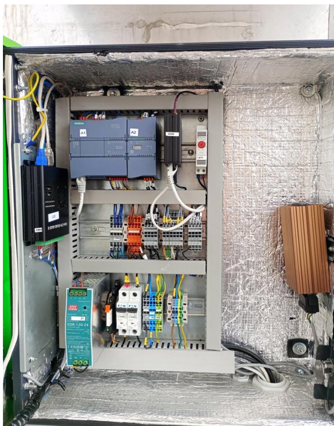
Wnętrze szafy sterującej systemem zrzutu ścieków dowożonych „Ścieki Polskie” po modernizacji.
