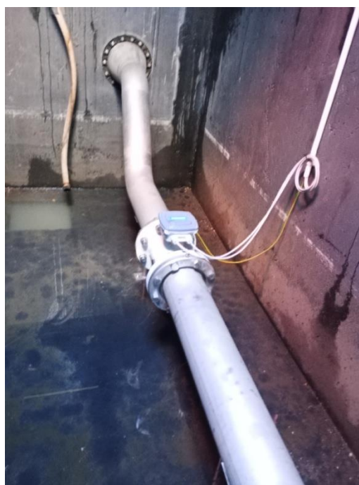
Sterownik przepływomierza Siemens SITRANS F M MAG 6000; zasyfonowany przepływomierz elektromagnetyczny SIEMENS DN 150 wraz z redukcją średnicy kolektora.
