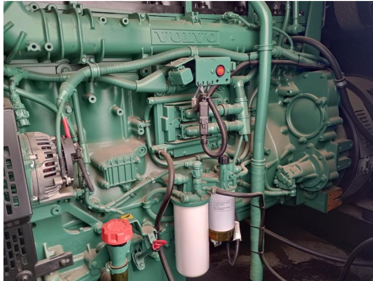
Silnik agregatu VOLVO PENTA GV 450 S.
